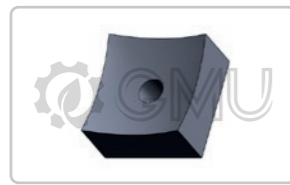
Nóż koronowy 42x42x22 M12 PC 4-FA BANO
